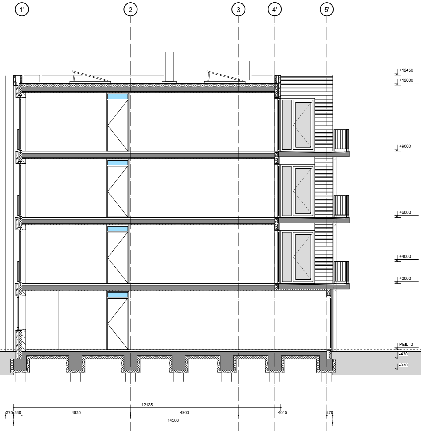
doorsnede A-A
