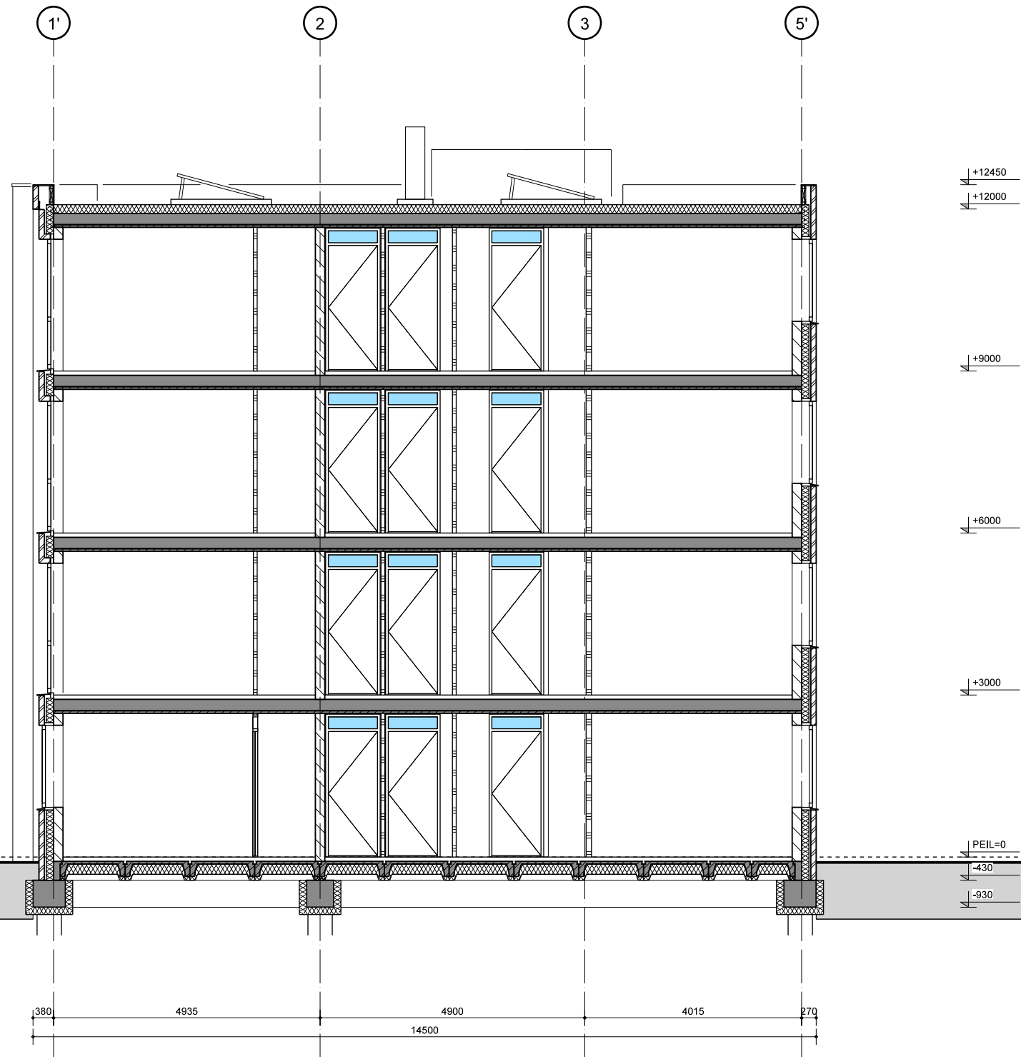
doorsnede B-B
